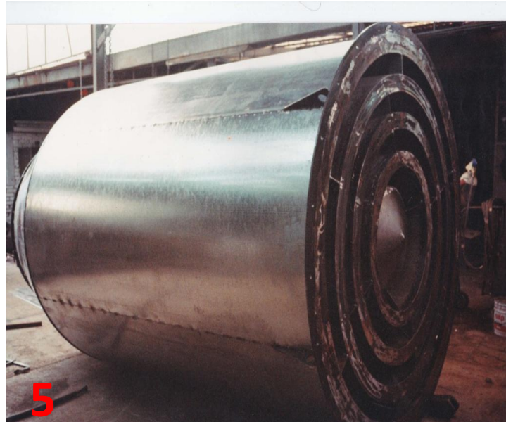
Alcuni degli interventi progettati e prodotti: Cabine Fonoisolanti per Mulini e Presse (1-6) Silenziatori d'Aria (3-5) Trattamento Ambientale (2) Cabina "riposo acustico uomo" (4)
